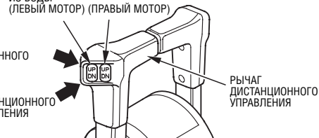
(тип R3) Пост управления спаренными подвесными моторами
