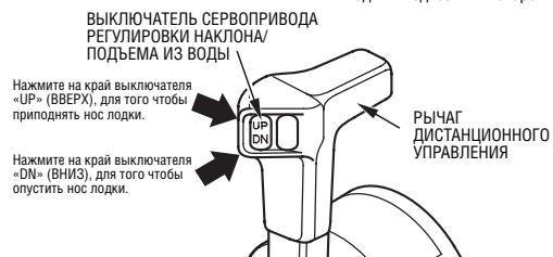
(тип R3) Пост управления спаренными подвесными моторами
